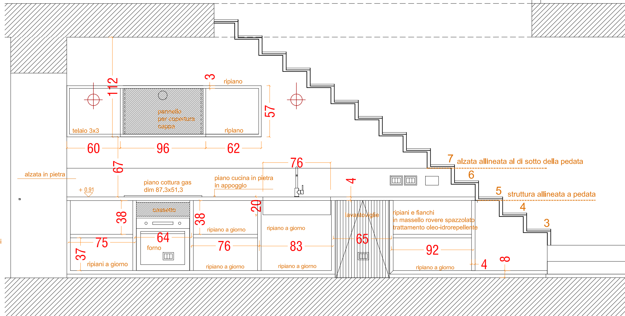
PROSPETTO
