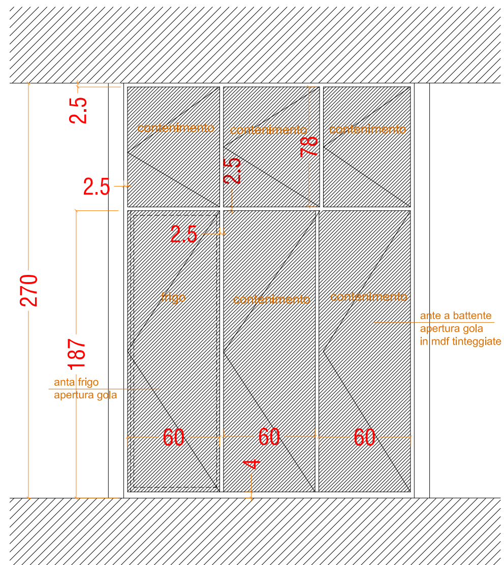
PROSPETTO ANTE
