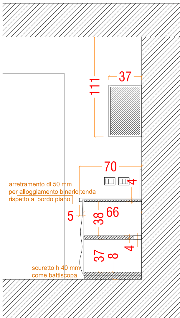
SEZIONE AA
