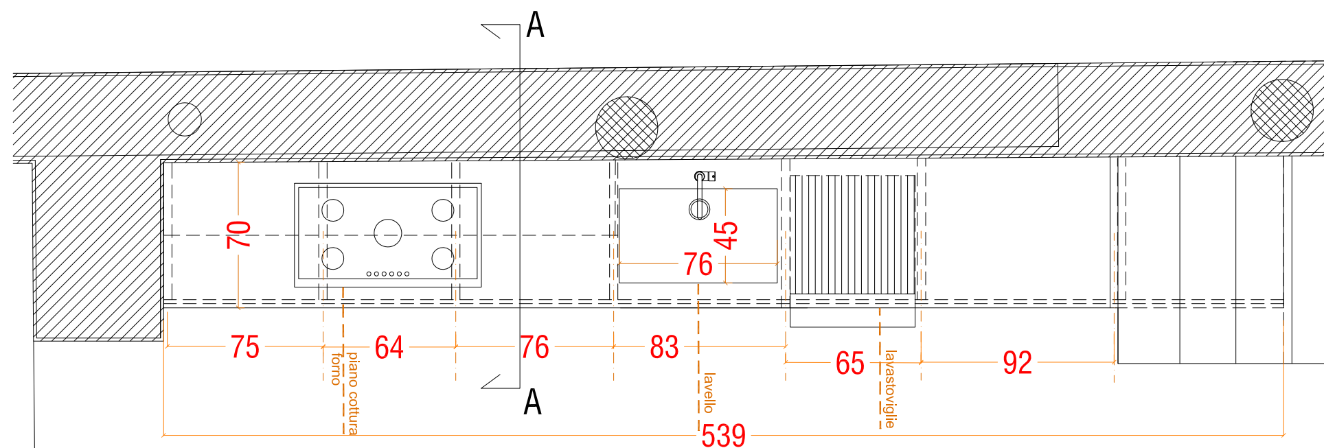
PIANTA
